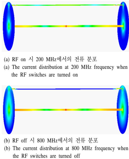
그림 2. 제안된 안테나의 전류 분포 Fig. 2. The current distribution of the proposed antenna.
