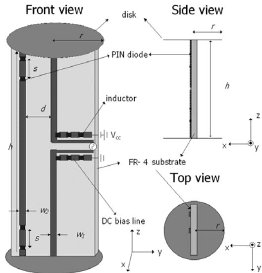
그림 1. 제안된 안테나 구조 Fig. 1. The proposed antenna structure.
