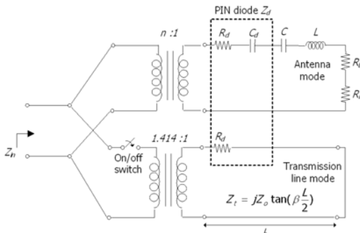
그림 8. 제안된 안테나의 등가 회로 모델 Fig. 8. The equivalent circuit model of the proposed antenna.
