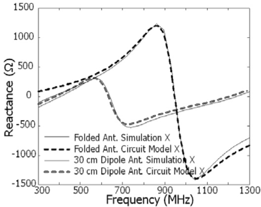
(b) 고주파 대역 입력 리액턴스 (b) The input reactance in high frequency band
